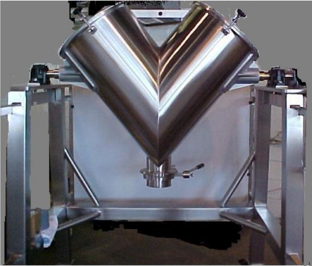
V-SHELL BLENDER
